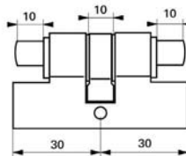
Cylindre profilé avec triangle interne
