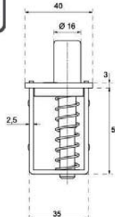
Gond à dé clic rapide, partie supérieure
