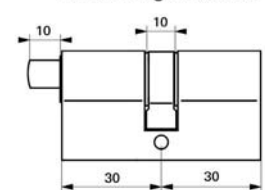
Cylindre profilé avec triangle externe
