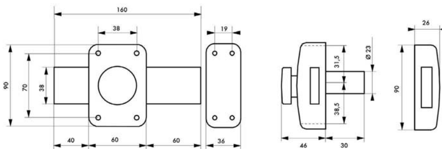
Foncet vissé démontable
