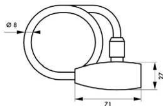
Longueur de câble : 1,50 m
