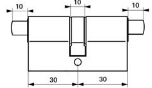
Cylindre profilé avec triangle externe
