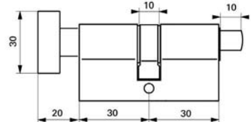
Cylindre profilé bouton avec triangle externe
